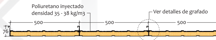
Poliuretano inyectado densidad 35 - 38 kg/m3
